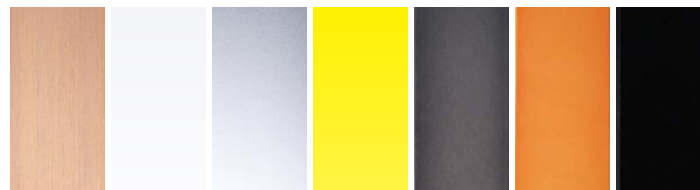
Größe/Dimensions/Dimensiones: 25x5x7 cm Gewicht / Weight / Peso: 0,250 KG Leuchtmittel/Bulbs/Bombillas: E27 max. 60 Watt
